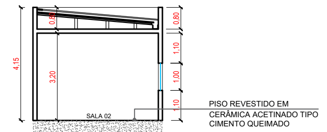
CORTE GG ESCALA 1/100
