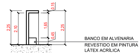
CORTE DD ESCALA 1/100
