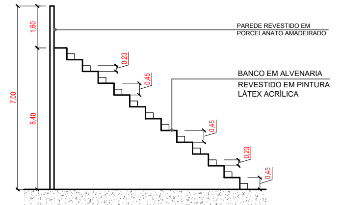
CORTE CC ESCALA 1/100
