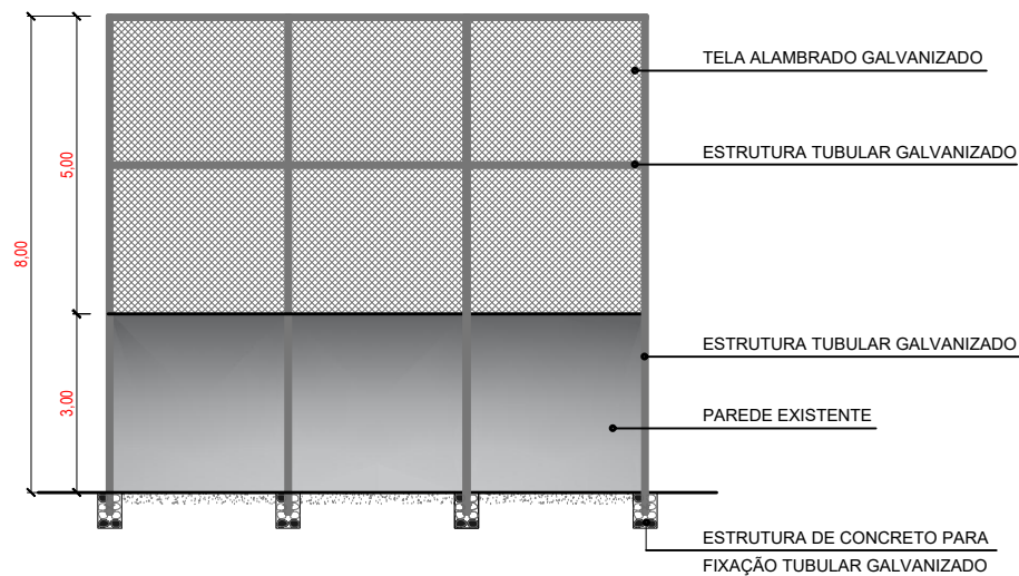
ELEVAÇÃO FRONTAL ESCALA 1/100
